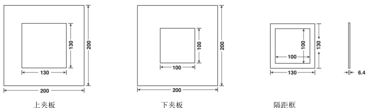
图3 试样夹持架
